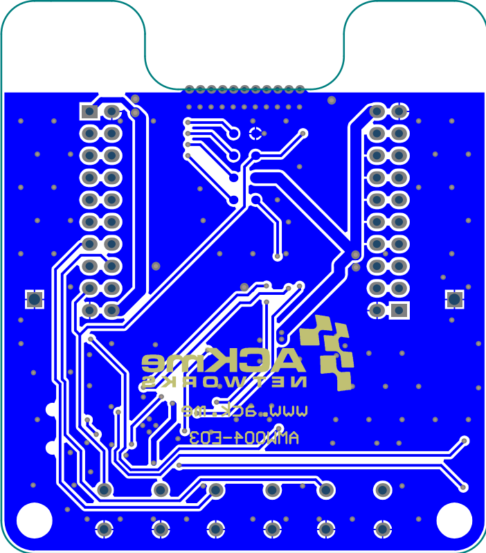
Bottom Layer
