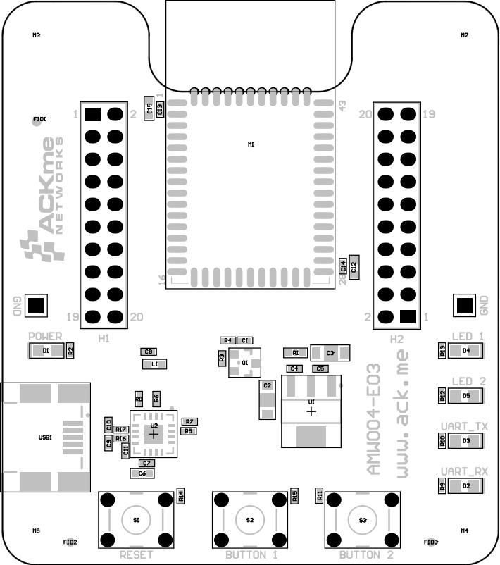
Top Overlay
